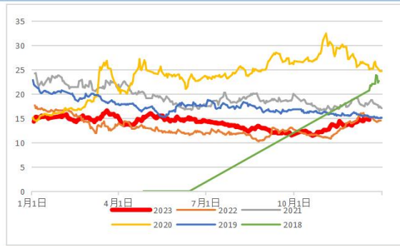
L/SC季节性
