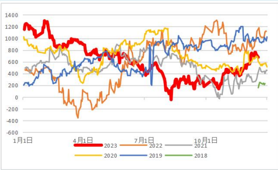
BU-FU季节性
