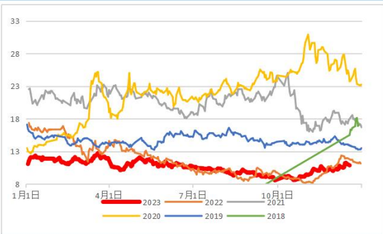
V/SC季节性
