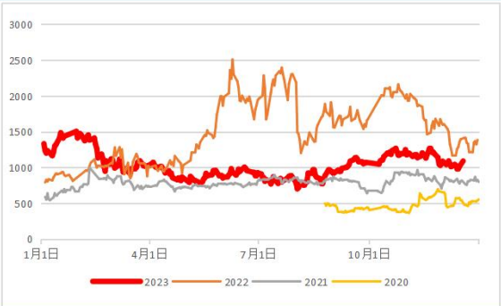
LU-FU季节性
