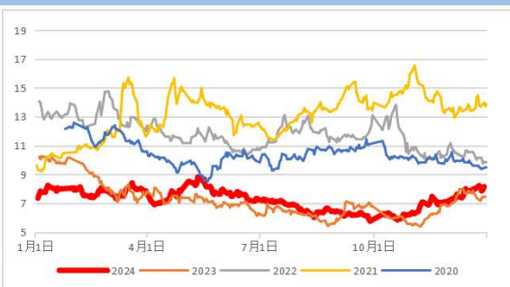
EG/SC季节性
