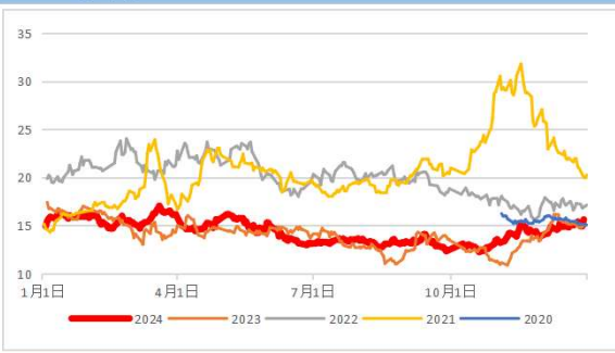
EB/SC季节性
