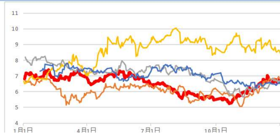
BU/SC季节性
