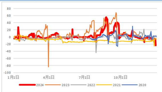
Sc_C1-C2季节性
