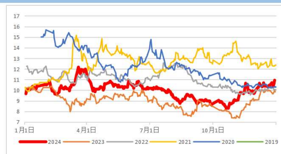
TA/SC季节性
