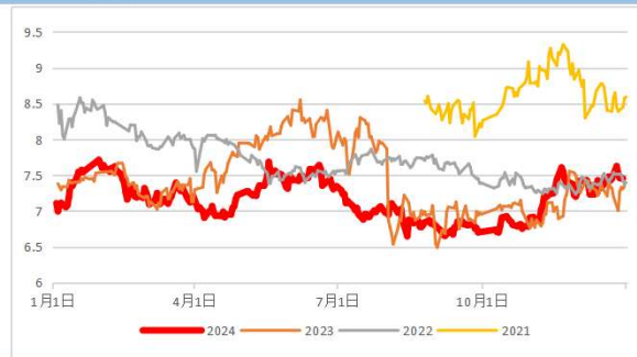
LU/SC季节性
