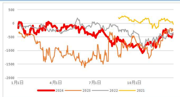
BU-LU季节性
