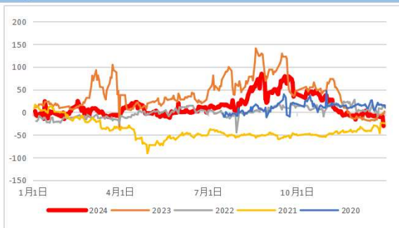
Sc_C1-C6季节性
