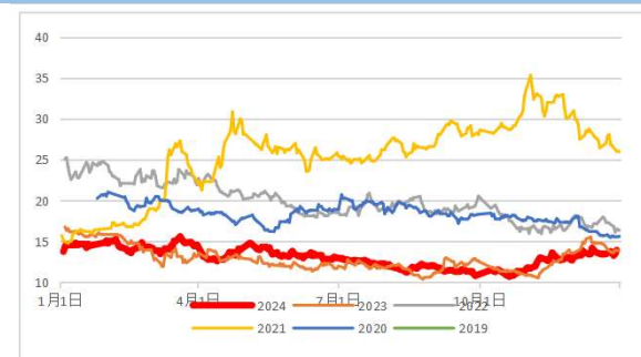
PP/SC季节性
