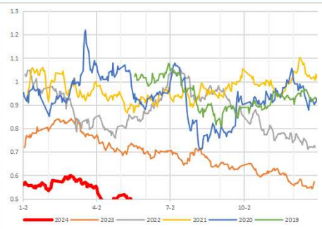
000300/Au季节性
