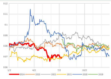
Au/Ag季节性
