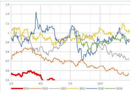
000300/Au季节性
