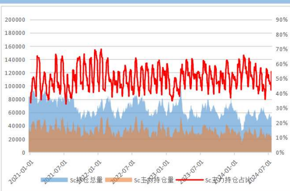
Sc持仓量
