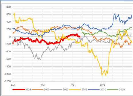
J-Jm季节性
