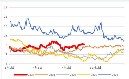
EG/SC季节性
