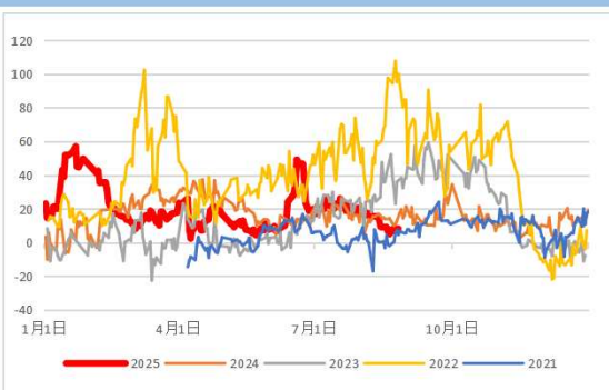
Sc_C2-C6季节性
