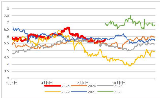
FU/SC季节性
