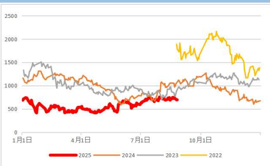
LU-FU季节性
